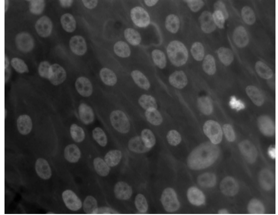
(d) \gamma = 0.5 .
