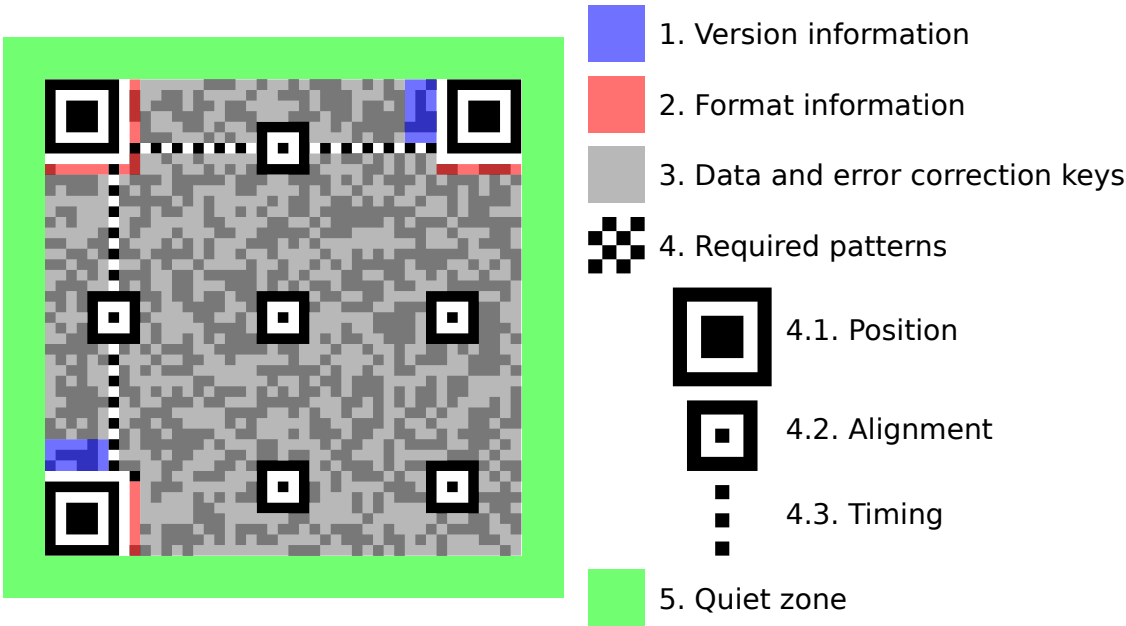
(b) Code.
