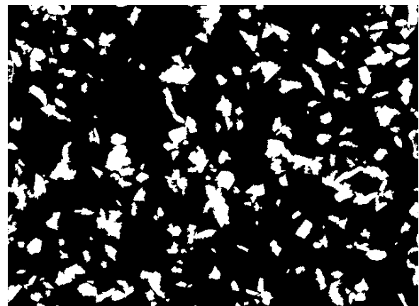
(d) Derivative.
