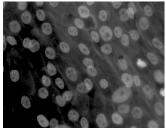
(d) \gamma = 0.5 .
