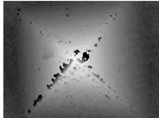
(d) Altitudes.
