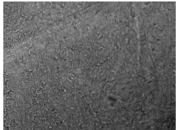
(d) Layer 24
