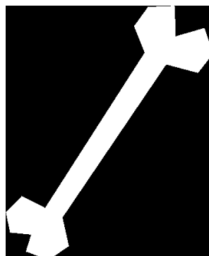
(b) Bone.
