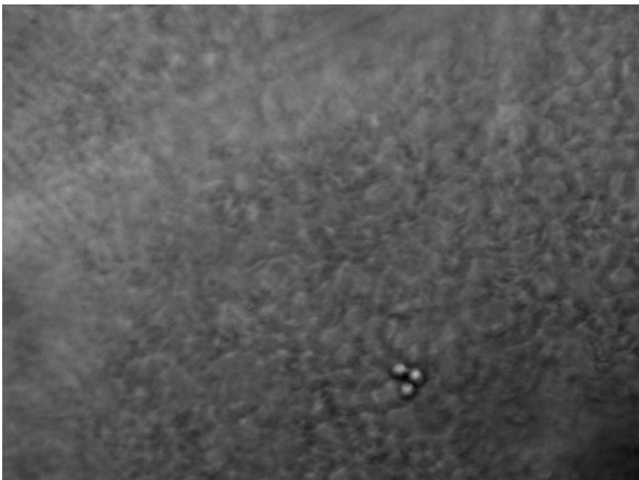
(c) Layer 18
