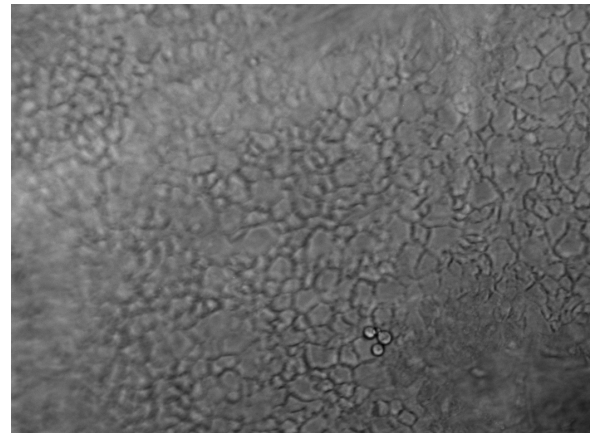
(d) Layer 24
