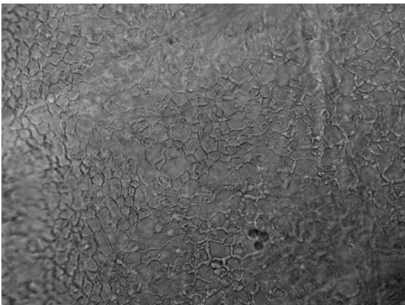
(c) Layer 18
