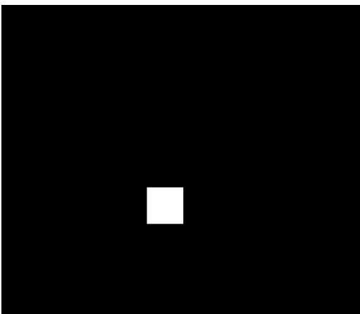
(a) ROI.
