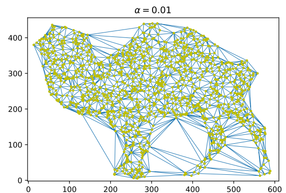
(d) \alpha = 1/100 .
