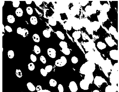
(d) E = 1000 .
